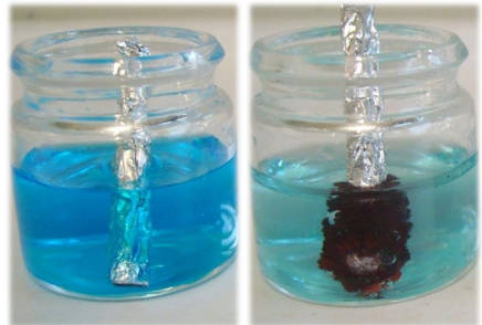
Verhalten von Aluminium in verd. Kupfersulfat-Lösung (links) und in verd. Kupferchlorid-Lösung (rechts)
