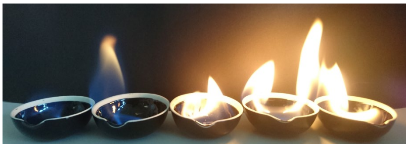
Flammenfärbung der Alkohole (von links nach rechts: Methanol, Ethanol, Propanol, Butanol, Pentanol)
